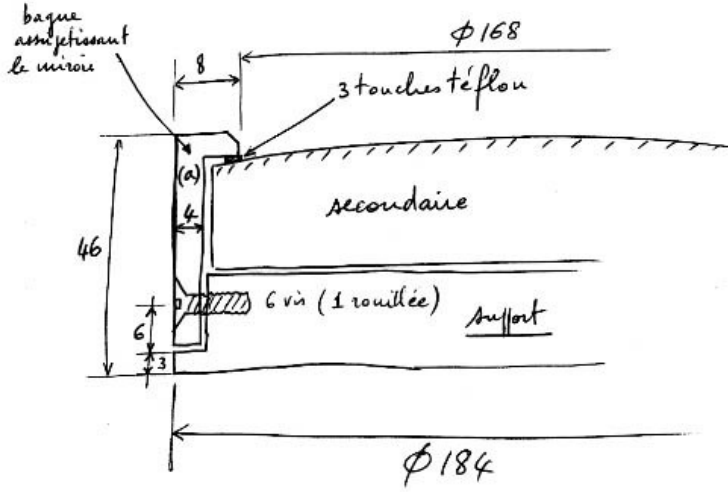
Barillet du miroir secondaire (b)
